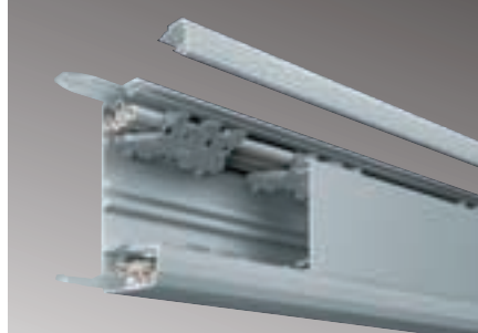
BR netway® z aluminium, pokrywa boczna
